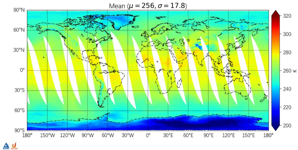
图 6-1 2024 年 5 月 13 日的 MWRI-II L1 模拟数据图（升轨）
