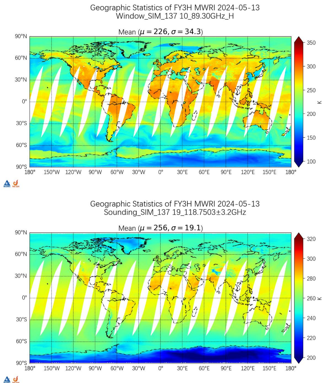
图 6-2 2024 年 5 月 13 日的 MWRI-II L1 模拟数据图（降轨）
